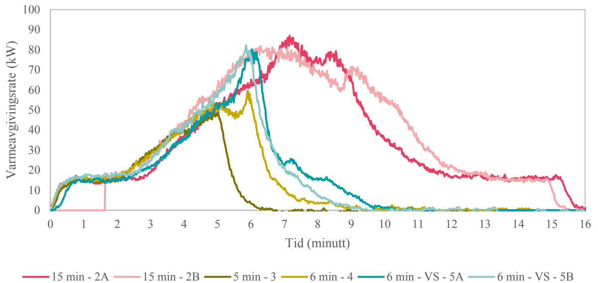
Figur 4-7: Varmeavgivingsrate for forsøk med einssidig glas, 6 cm holrom, 15 kW effekt på brennaren og ulik tid til brennaren vart slått av og to forsøk med vindsperre (VS 5A og 5B) vist med blå kurver.
