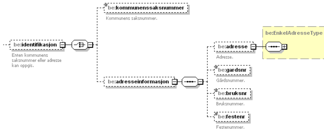
Figure 93 'identifikasjon' within ProsjektType
