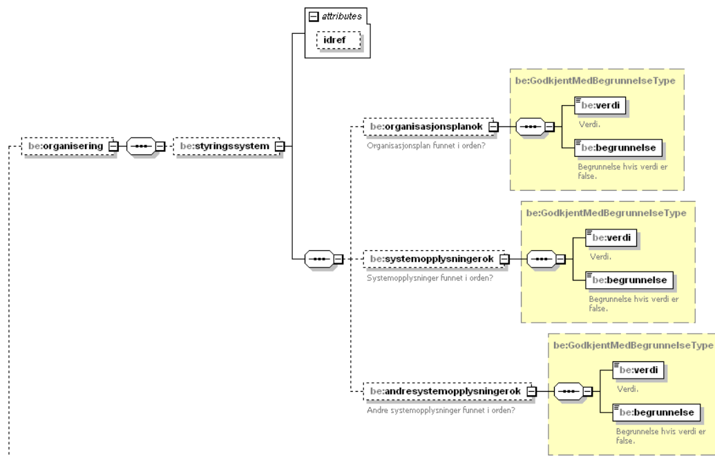
Figure 9 Element structure 'organisering' within 'saksbehandling' in 'sentralgodkjenning'
