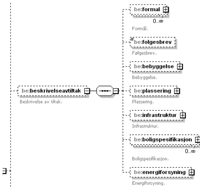
Figure 29 Element structure 'beskrivelseavtiltak' under 'sak' in 'byggesak'
