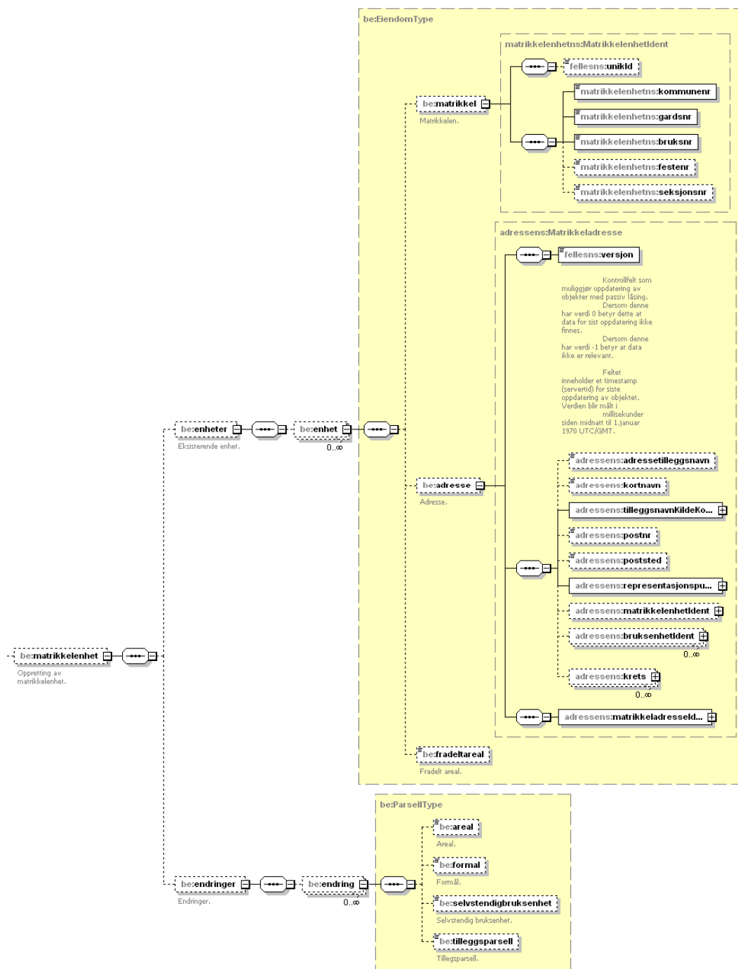
Figure 23 Element structure 'matrikkelenhet' under 'sak' in 'byggesak'
