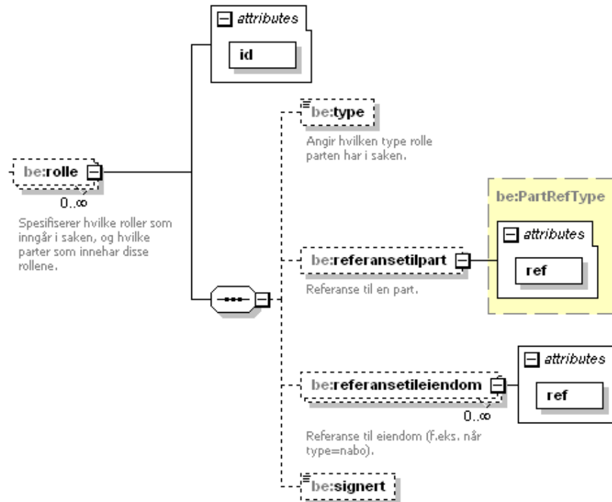
Figure 39 Element structure 'rolle' under 'sak' in 'byggesak'
