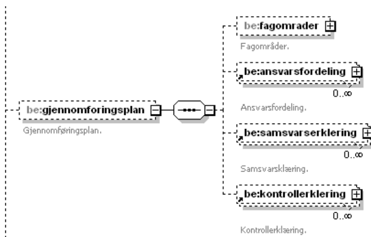
Figure 41 Element structure 'gjennomforingsplan' under 'sak' in 'byggesak'
