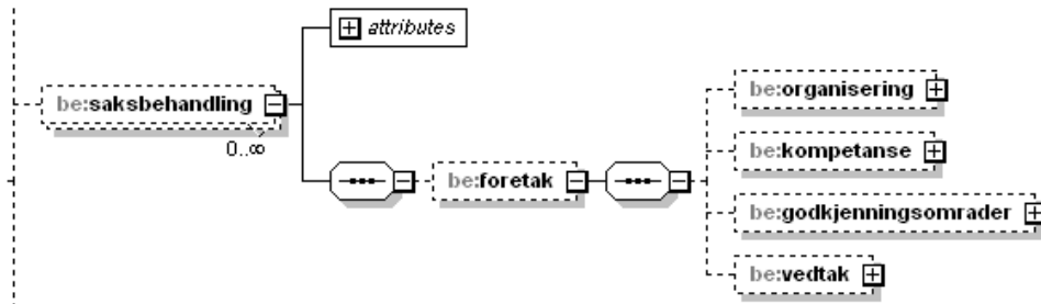
Figure 8 Element structure 'saksbehandling' within 'sentralgodkjenning'.
