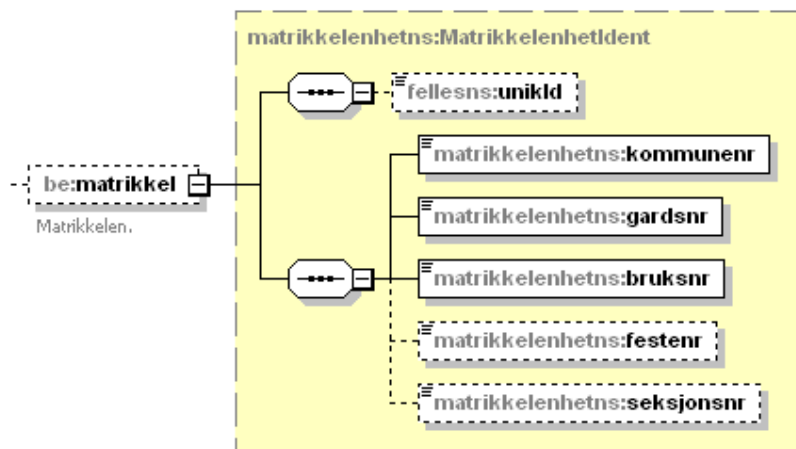
Figure 68 Complex type matrikkelenhets:Matrikkelenhet
