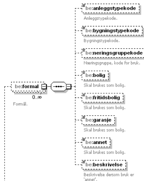
Figure 30 Element structure 'formal' under 'beskrivelseavtiltak' in 'byggesak'
