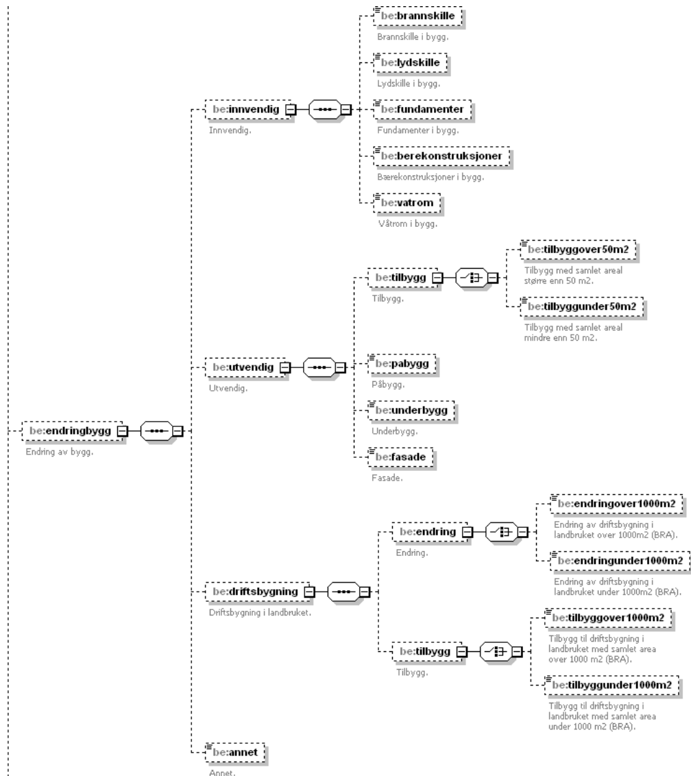
Figure 100 "endringbygg" within TiltakType
