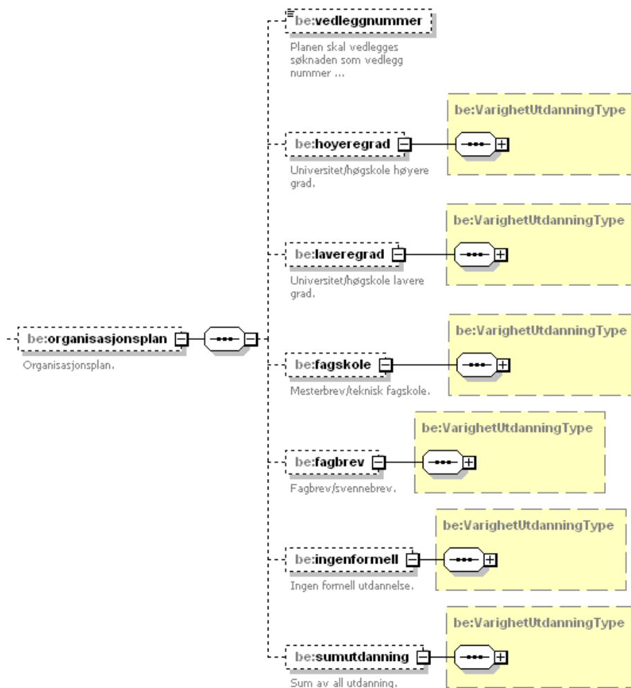
Figure 84 'organisasjonsplan' within OrganisererType
