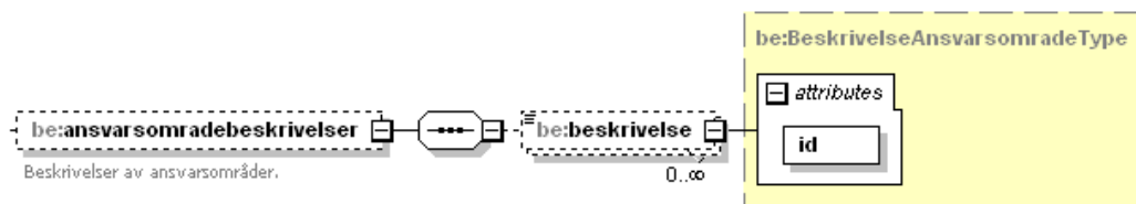
Figure 40 Element structure 'ansvarsomradebeskrivelser' under 'sak' in 'byggesak'
