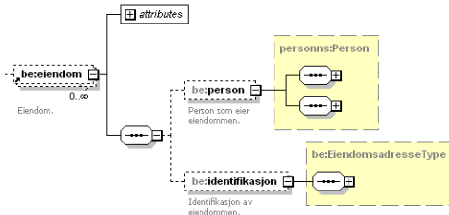
Figure 37 Element structure 'eiendom' under 'sak' in 'byggesak'
