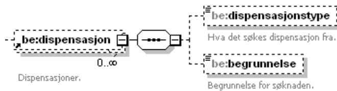
Figure 36 Element structure 'dispensasjon' under 'sak' in 'byggesak'
