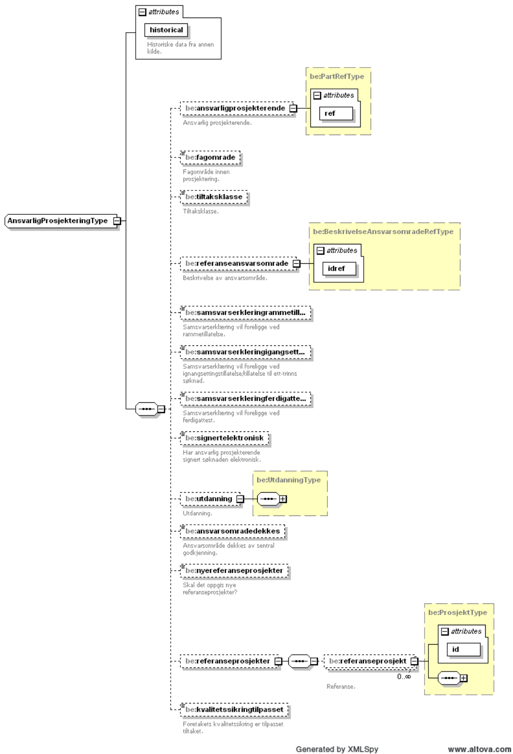
Figure 60 Complex type AnsvarligProsjekteringType
