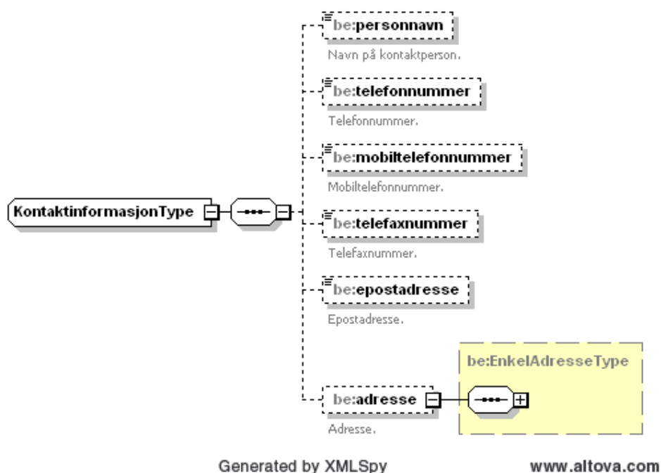
Figure 79 Complex type KontaktinformasjonType
