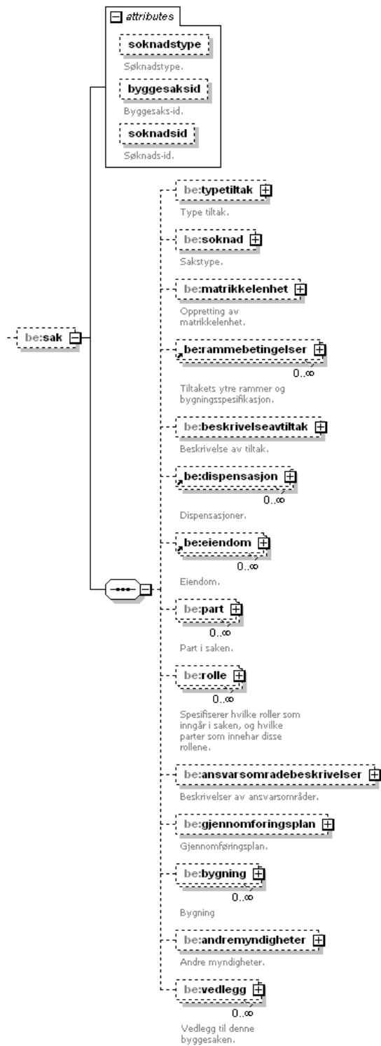
Figure 16 Element structure 'sak' within 'byggesak'
