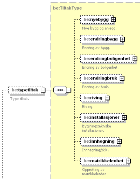
Figure 17 Element structure 'typetiltak' within 'sak' in 'byggesak'
