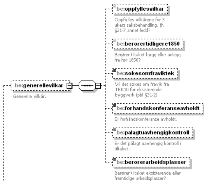
Figure 25 The element structure 'generellevilkar' under 'rammebetingelser' in 'byggesak'
