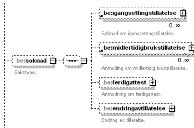
Figure 18 Element structure 'soknad' within 'sak' in 'byggesak'
