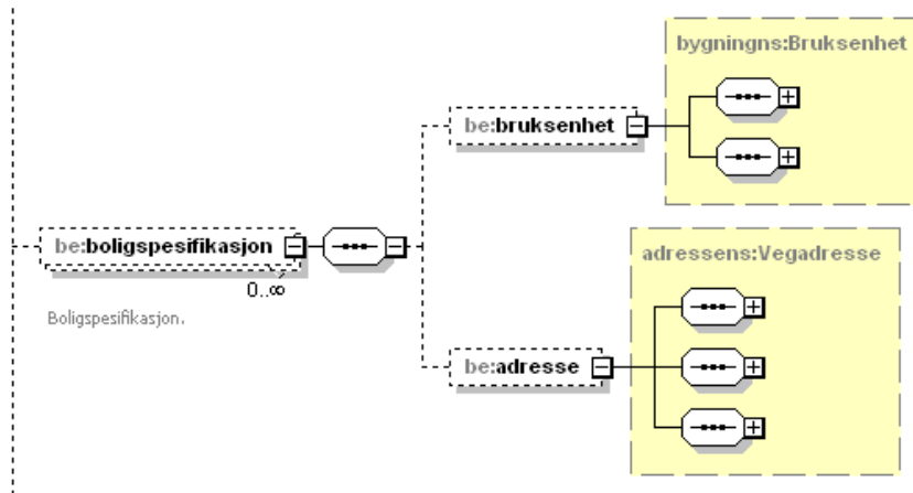
Figure 34 Element structure 'boligspesifikasjon' under 'beskrivelseavtiltak' in 'byggesak'
