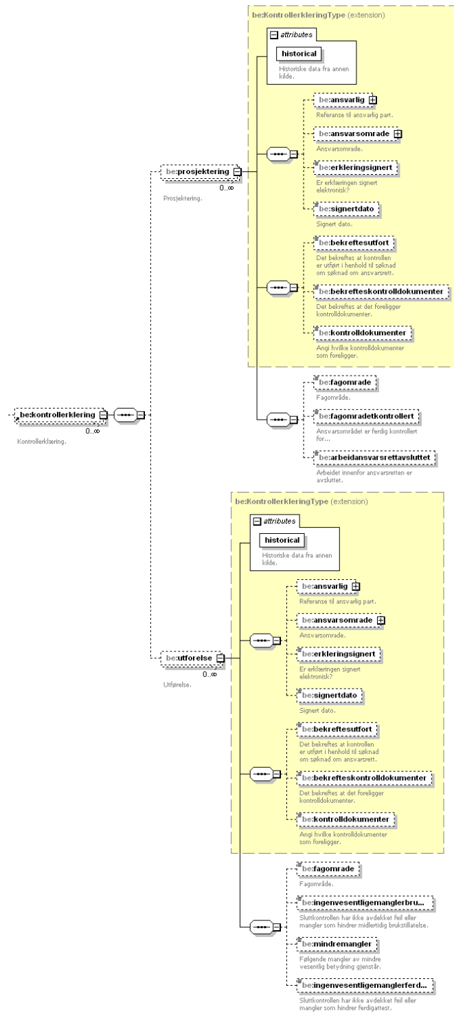
Figure 45 Eement structure 'kontrollerklæring' under 'gjennomforingsplan' in 'byggesak'
