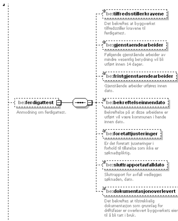
Figure 21 Element structure 'ferdigattest' under 'soknad' in 'byggesak'
