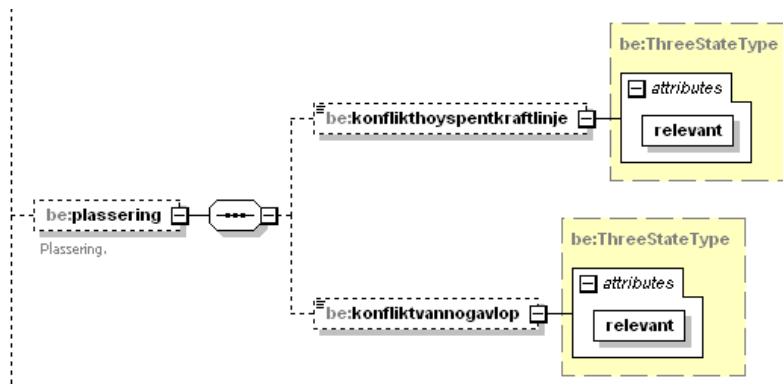
Figure 32 Element structure 'plassering' under 'beskrivelseavtiltak' in 'byggesak'
