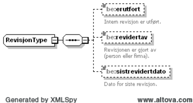
Figure 95 Complex type RevisjonType
