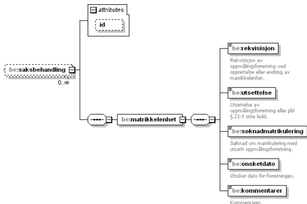
Figure 49 Element structure 'saksbehandling' under 'byggesak'
