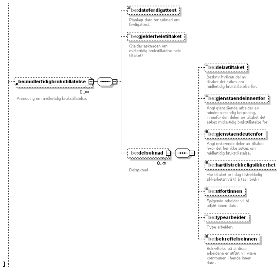
Figure 20 Element structure 'midlertidigbrukstillatelse' under 'sak' in 'byggesak'
