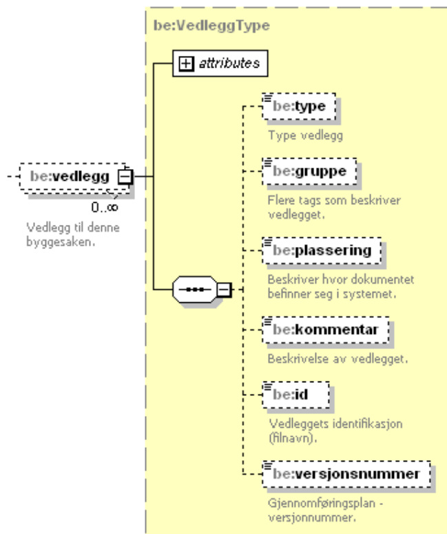
Figure 48 Element structure 'vedlegg' under 'sak' in 'byggesak'
