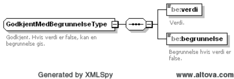
Figure 77 Complex type GodkjentMedBegrunnelse
