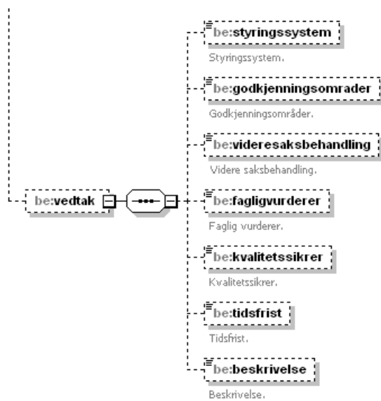
Figure 12 Element structure 'vedtak' within 'saksbehandling' in 'sentralgodkjenning'
