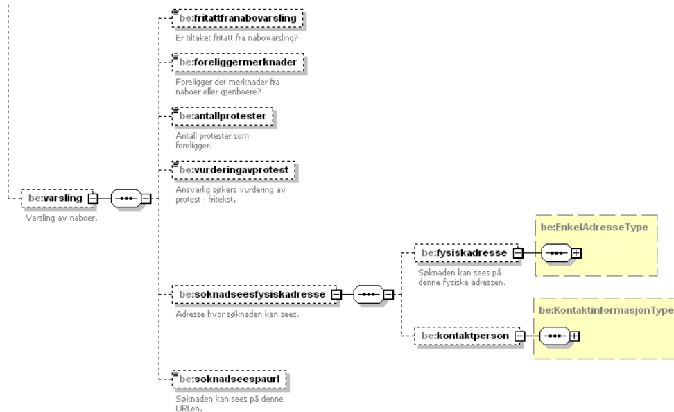
Figure 28 Element structure 'varsling' under 'rammebetingelser' in 'byggesak'
