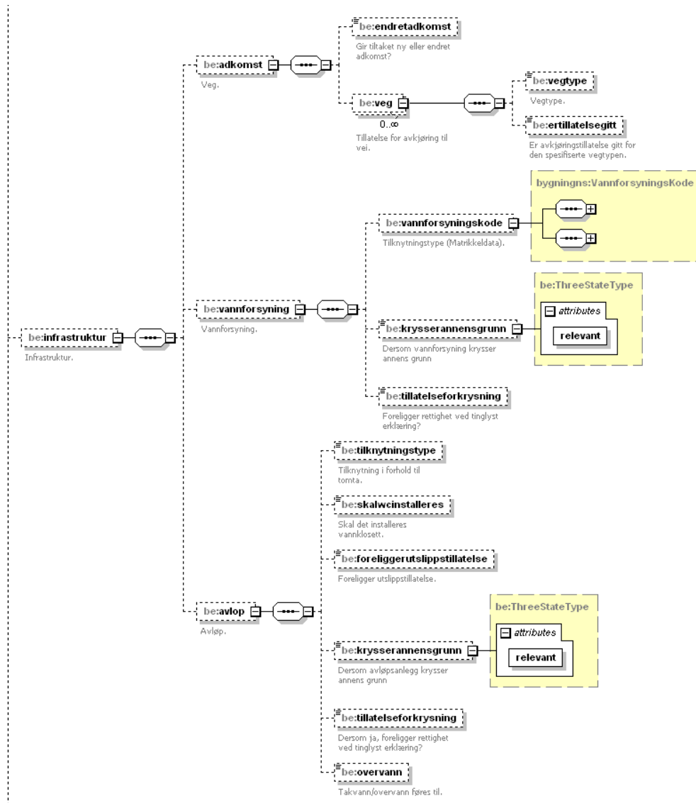
Figure 33 Element structure 'infrastructure' under 'beskrivelseavtiltak' in 'byggesak'
