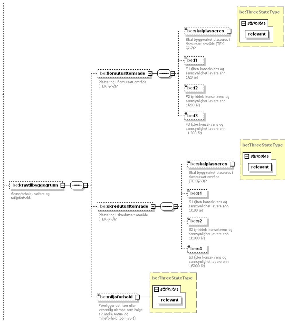
Figure 27 Element structure 'kravtilbyggegrunn' under 'rammebetingelser' in 'byggesak'
