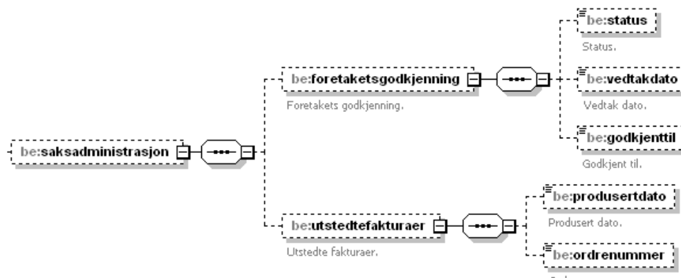
Figure 13 Element structure 'saksadministrasjon' within 'sentralgodkjenning'.
