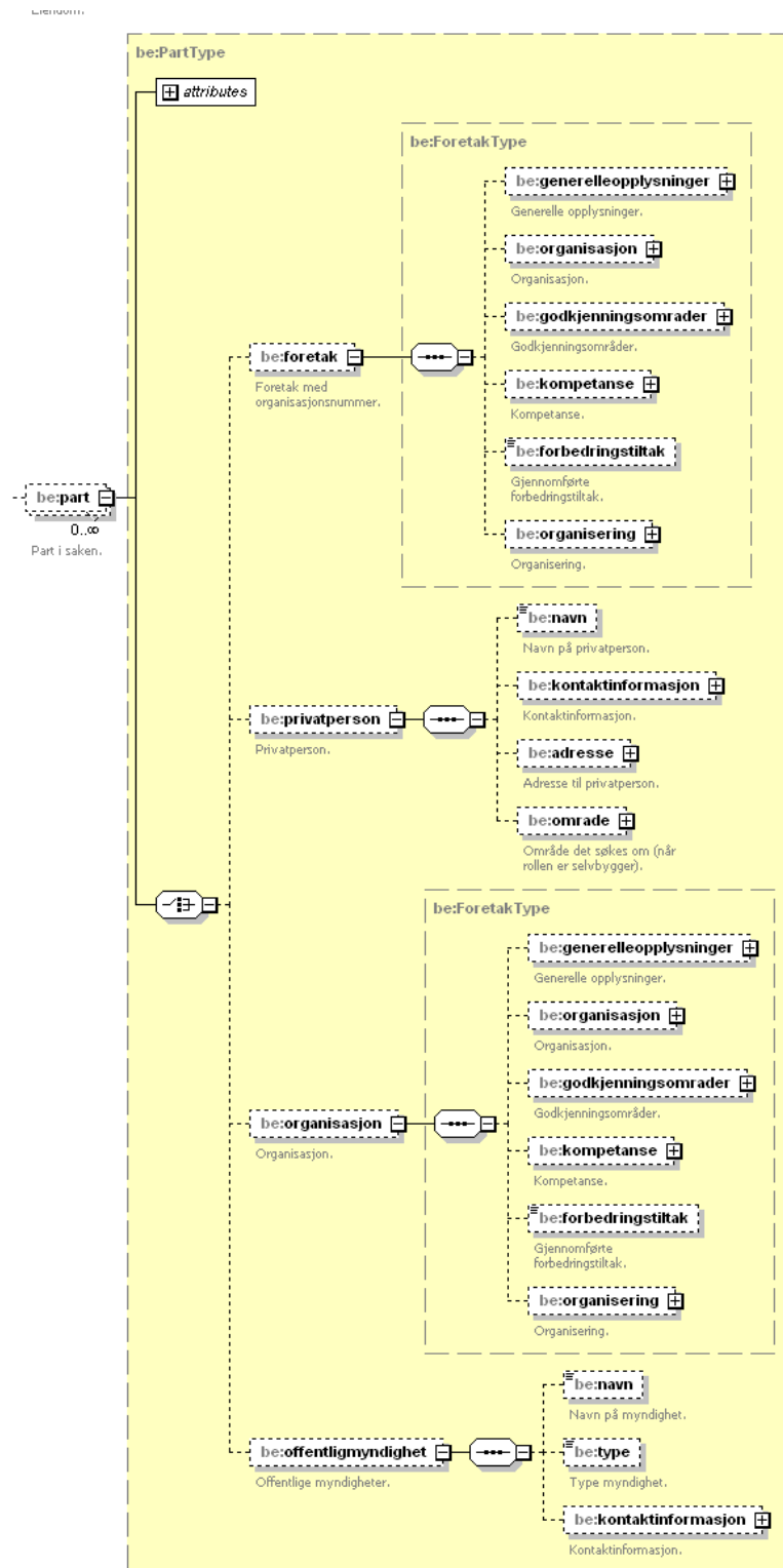
Figure 38 Element structure 'part' under 'sak' in 'byggesak'
