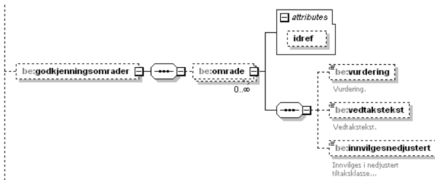
Figure 11 Element structure 'godkjenningsomrader' under 'saksbehandling' in 'sentralgodkjenning'
