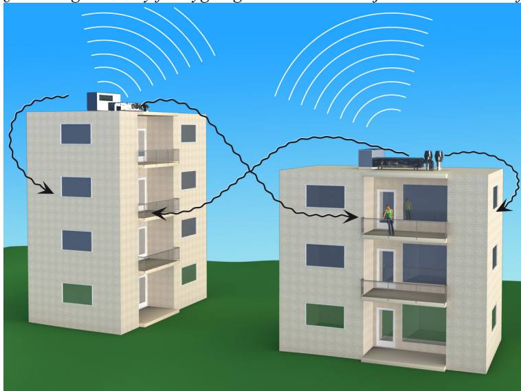
§ 13-9 Figur 1: Støy fra bygningstekniske installasjoner. Grenseverdi for utendørs maksimalt lydtryknivå.
